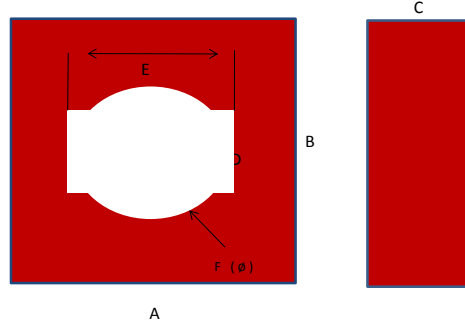
O.T.20 / O.T.30 / O.T.40 / O.T.60 / O.T.80 / O.T.100 / O.T.125 TRAFÖ ÖLÇÜLERİ
